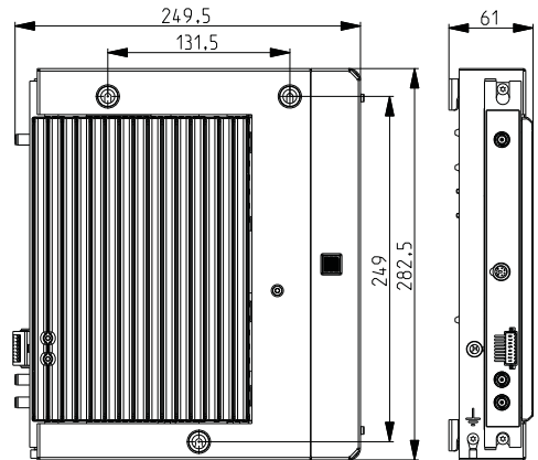
Abb. 2: Abmessungen und Montagepunkte
